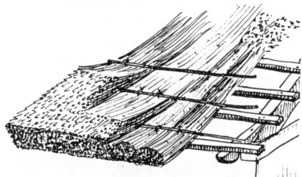
Princippet i bundne (kæppetækkede) tage.
